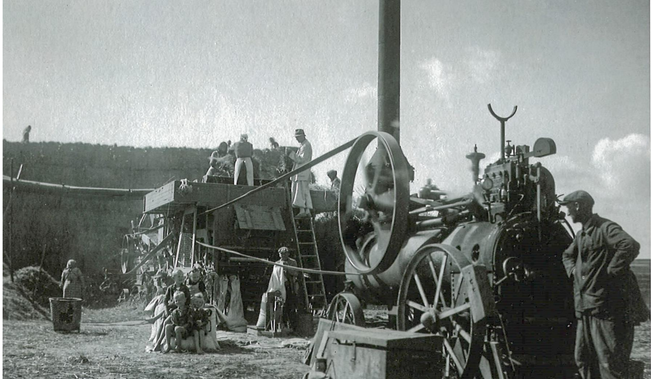
Lokomobila s mlátičkou
